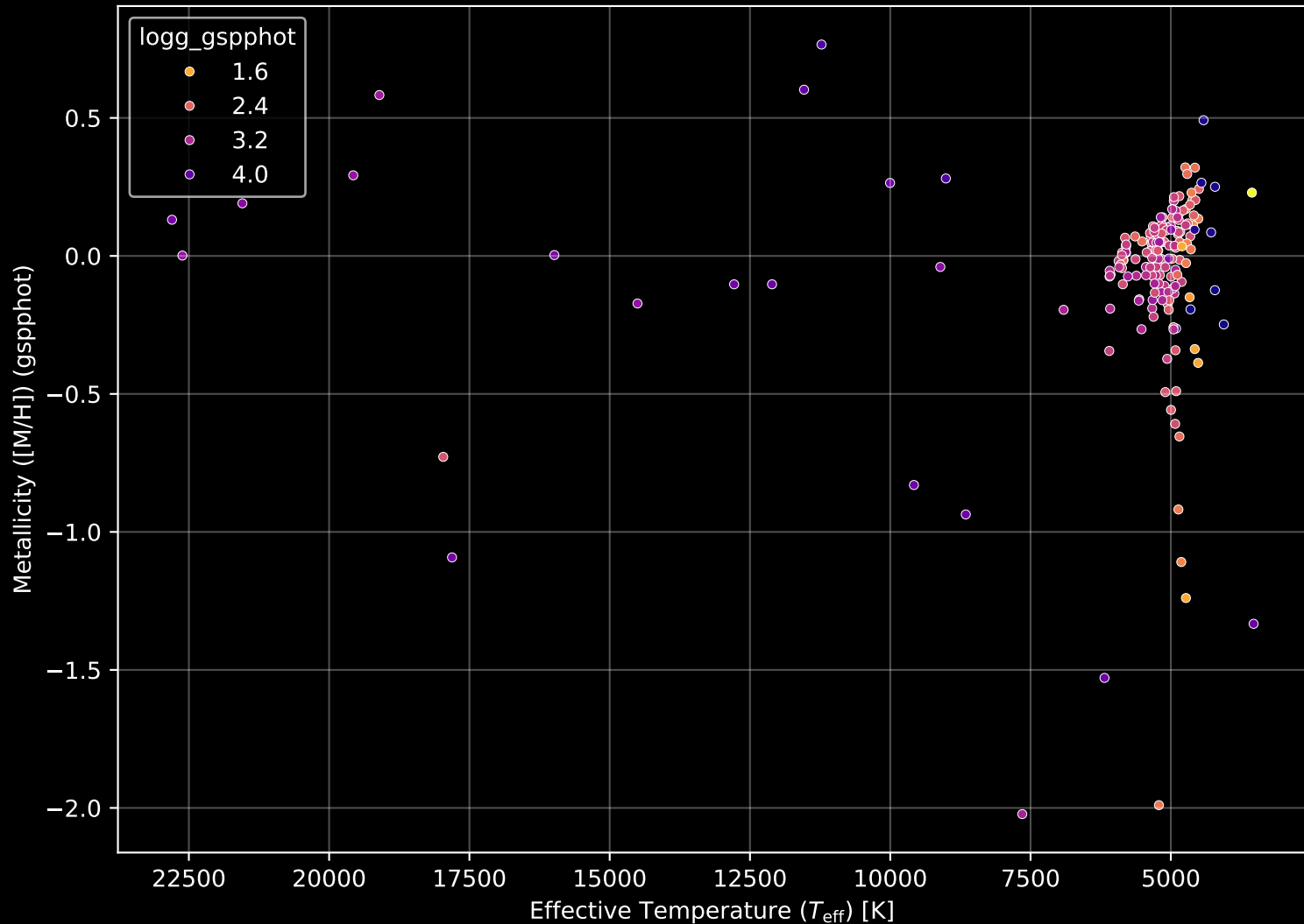
APOGEE DR17 Field: [146+04] Stellar Population Parameters (n= 197)
